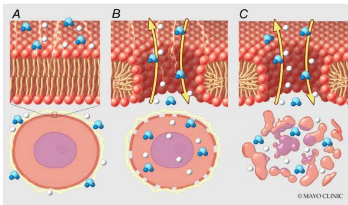
図3 : 高電圧をかけることで細胞の膜を破壊し、アポトーシスを誘導している様子
